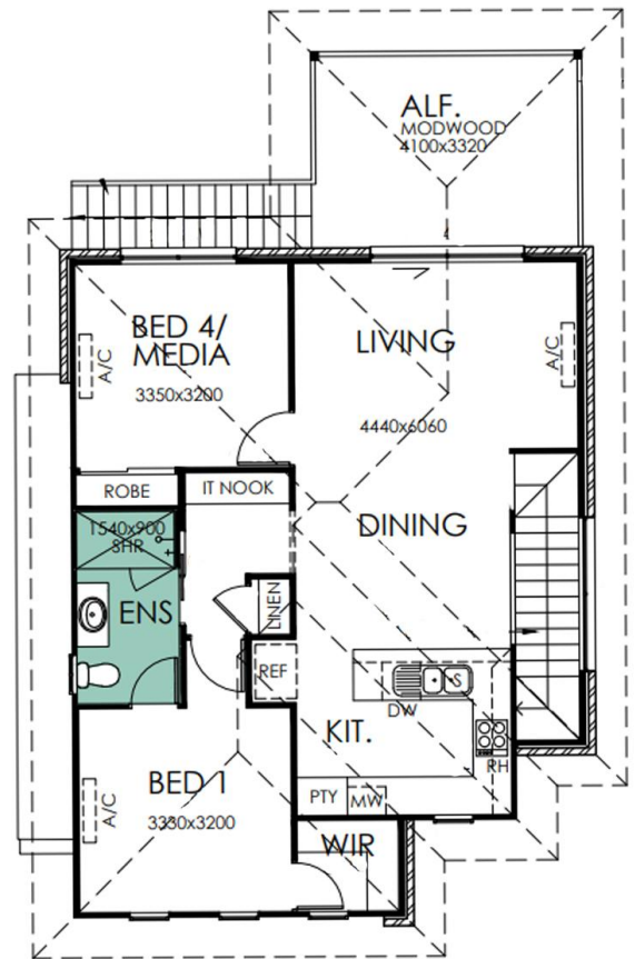
F/F PLAN
